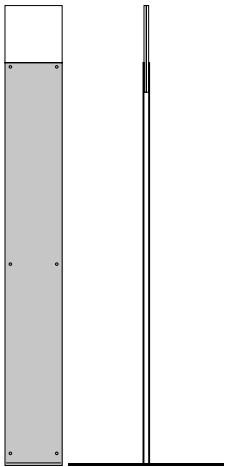
sil 304 VV SS w 180 x h 1448 x d 490mm w 7,09 x h 57,01 x d 19,29"
